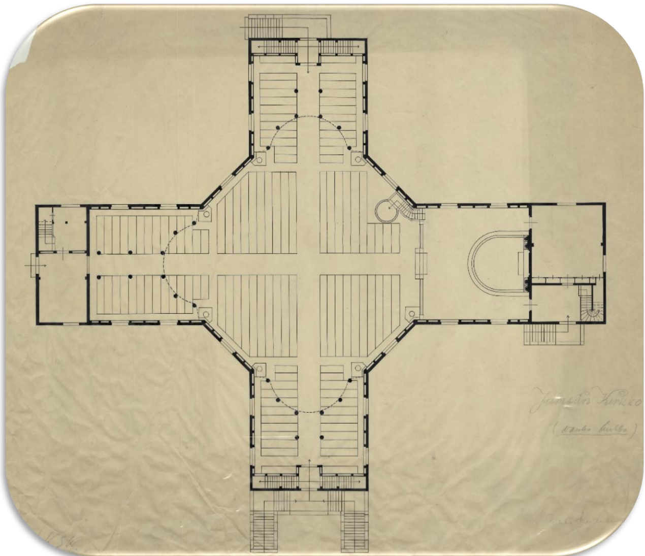
Kirkon pohjapiirros remontin jälkeen. Lähde: Kiianlehto, Sirkka. Aalto-yliopisto. Arkkitehtuurin mittauspiirrokset. ArkMP:1933_069.
